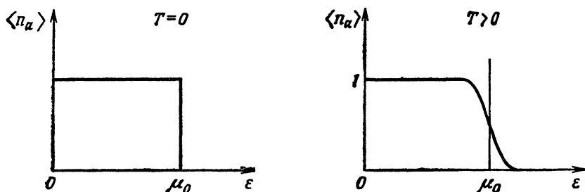
ФИГ. 1.8. Заполнение состояний при T=0 и при T>0 .
