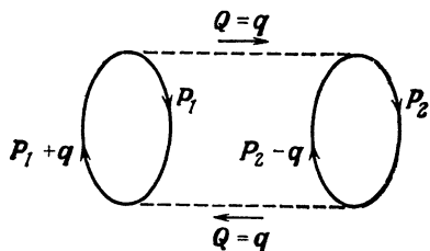
ФИГ. 9.8. Первая диаграмма на фиг. 9.5.
