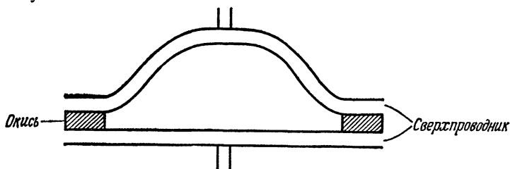
ФИГ. 10.30. Схема системы „с двумя щелями“.
