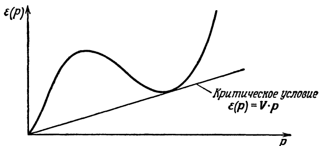
ФИГ. 11.23. Определение критической скорости. Критическая скорость определяется наклоном касательной к кривой \epsilon(p)
