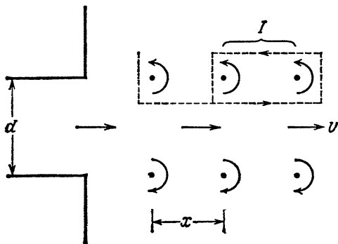
ФИГ. 11.32. Вихревые линии в жидкости, вытекающей из отверстия.
