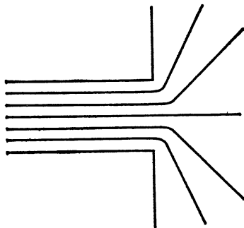
ФИГ. 11.31. Безвихревой поток из отверстия.
