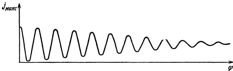
ФИГ. 10.29. Экспериментальное изменение j_{\text{макс}} .
