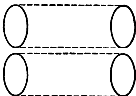
ФИГ. 9.7. Диаграмма четвертого порядка.
